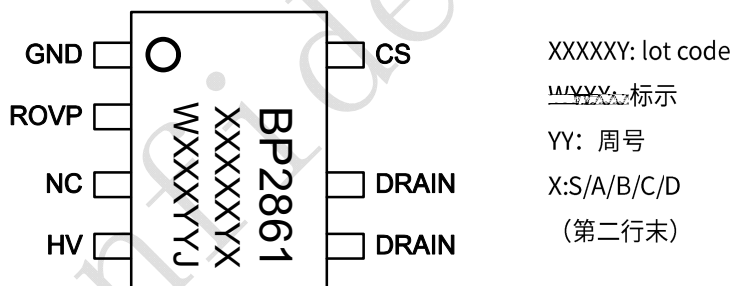
图 7 管脚封装图
